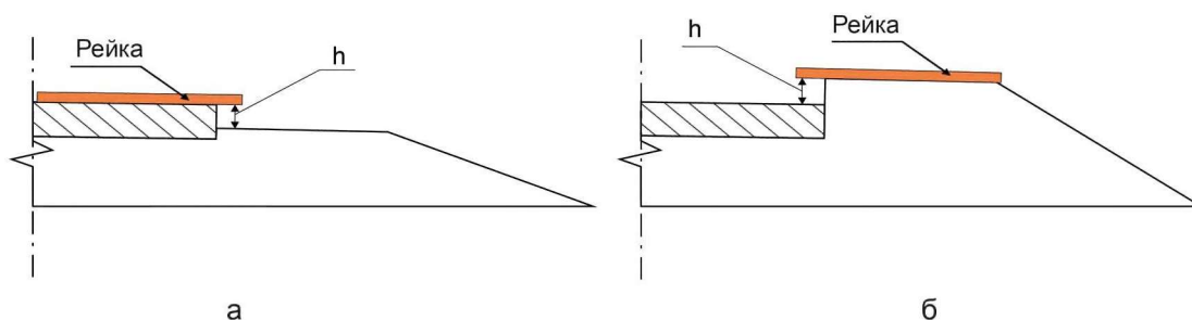
Рисунок 1 - Схема измерения величины занижения (возвышения) обочины и разделительной
